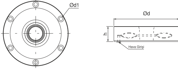
Ürün Nr. 1060 ER-EL Zero Clamp Gövde
