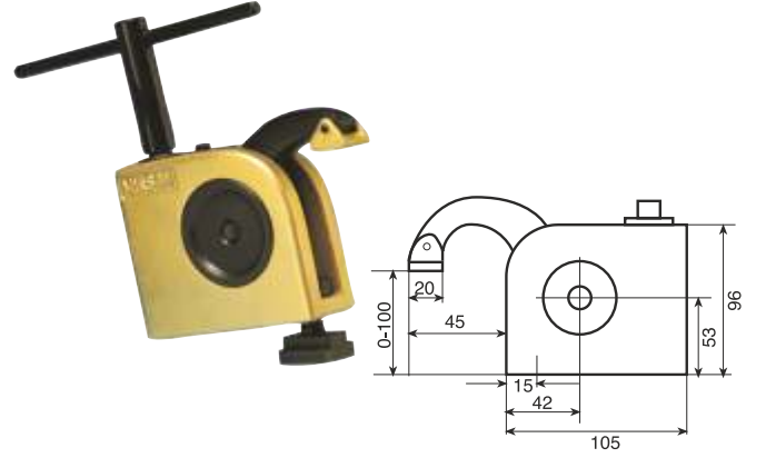
MFK 2042 Ağırlık : 800 gr. Genişlik : 40 mm.
