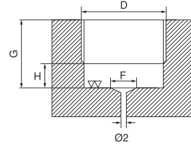
Bağlama Diyagramı Mounting Diagram
