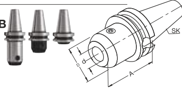
Mors Adaptörü DIN 6383
