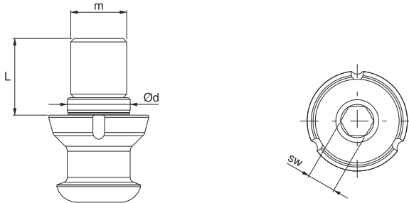
Ürün Nr. 1065 Çektirme Cıvatası
